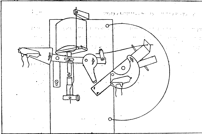
FIG. XVI. — MINUTERIE AVANT RÉENCLANCHEMENT.
