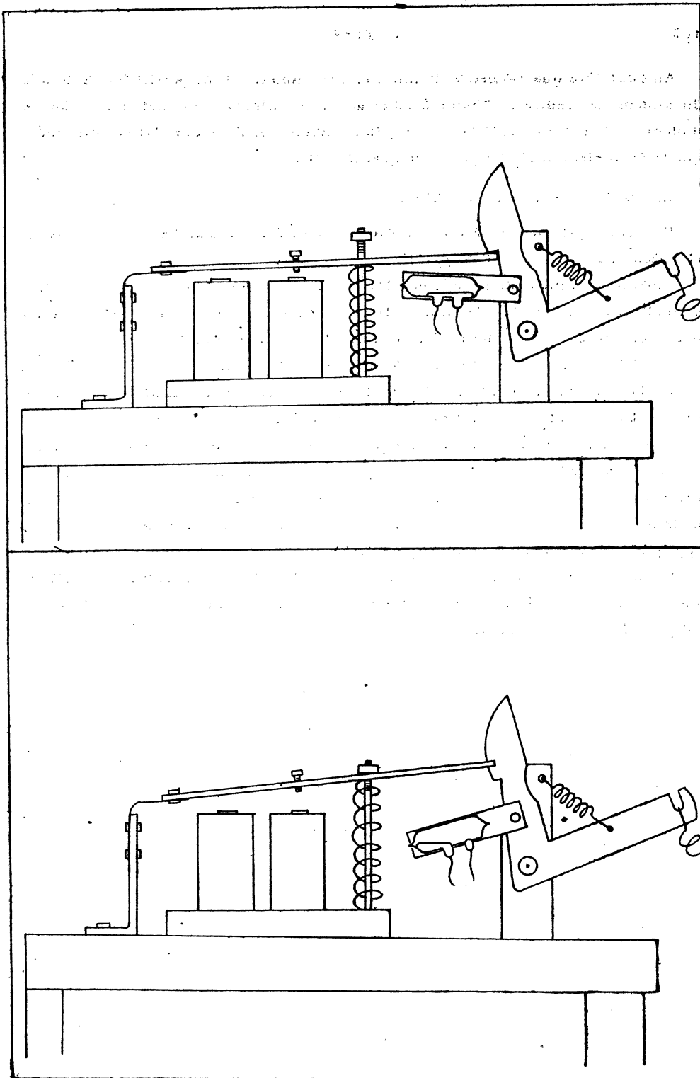
FIG. XIX. — COMMANDE DU MOTEUR DES GAMES; FONCTIONNEMENT.
