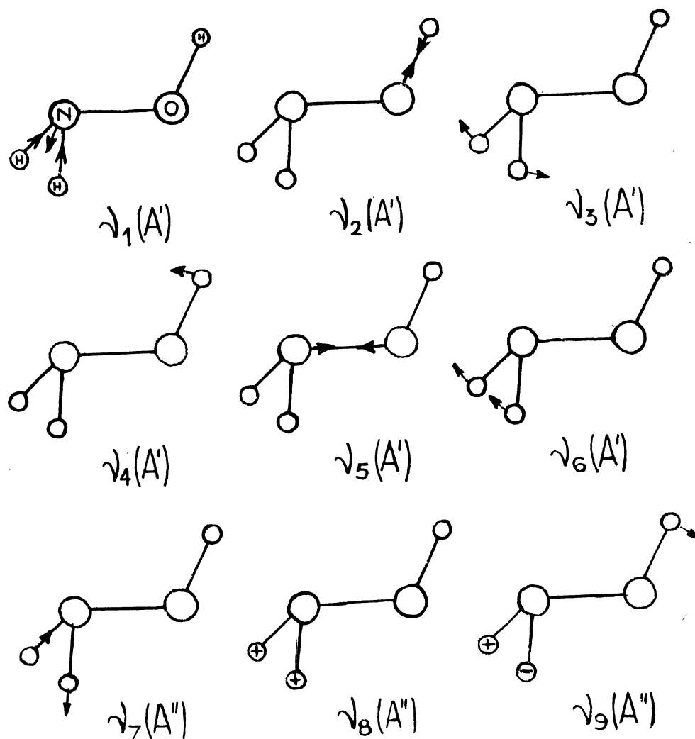
FIG. 1. — Modes de vibration de \text{NH}_2\text{OH} .
